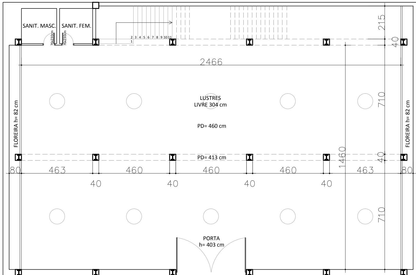
PLANTA SUBSOLO
